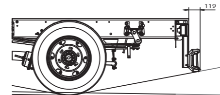
DETAIL FOR ARGENTINE VEHICLE Detalle para vehículo da Argentina
