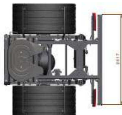
DETALHE PARA MERCADO ARGENTINA
