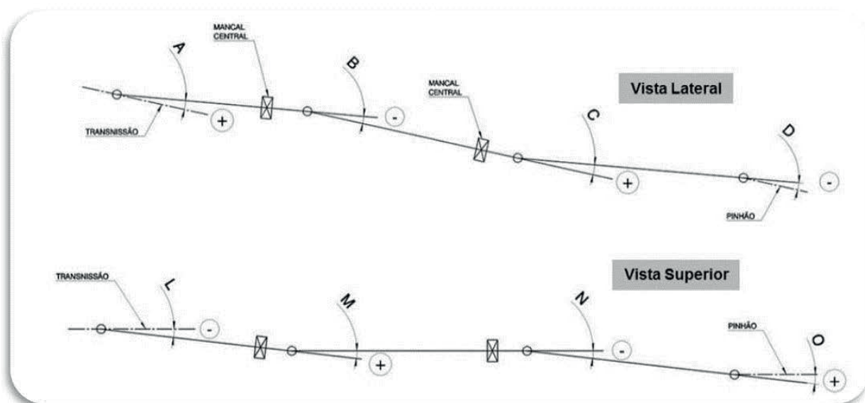
Diagrama de Ângulos
