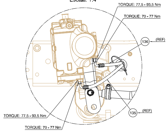
DETALHE B Escala: 1:4
