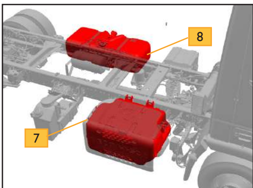
7 e 8 - HI-SCR e tanque de combustível
