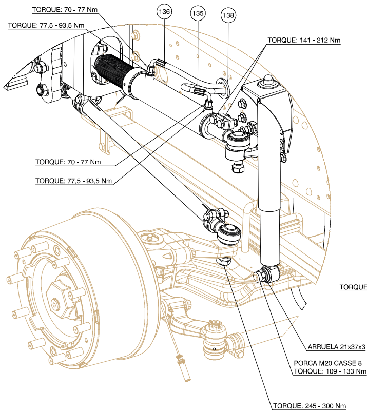
DETALHE A Escala: 1:4
