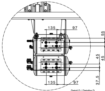
Detail D / Detalhe D
