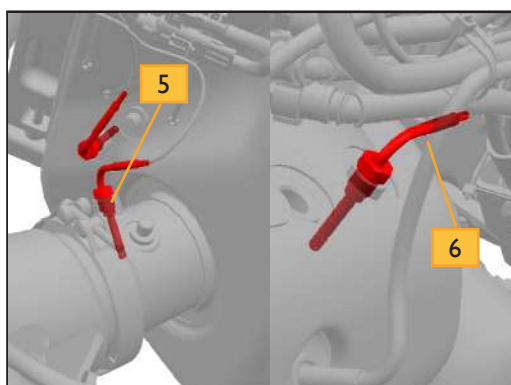
5 e 6 - Sensor de temperatura, entrada e saída de gases do escapamento e do catalisador
