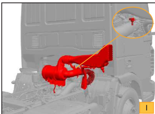
1 - Sensor de umidade no sistema de admissão do filtro de ar
